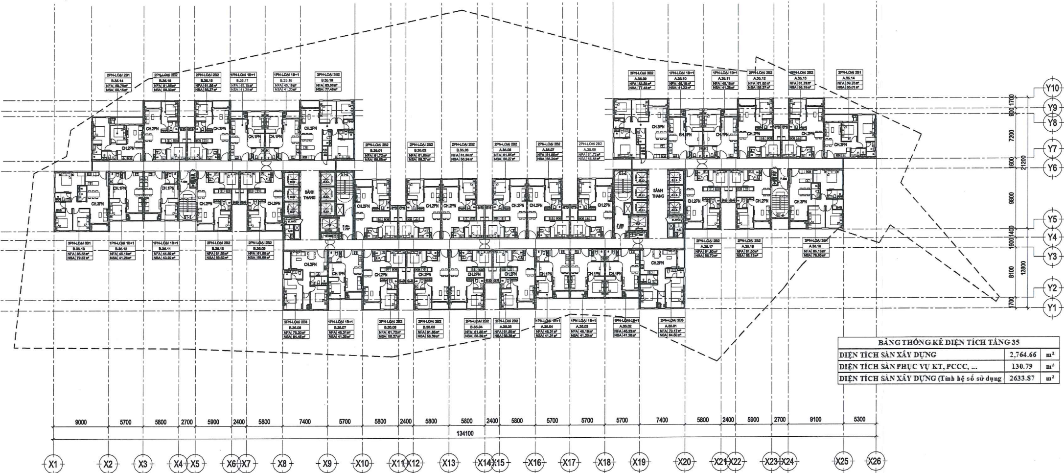
MẶT BẰNG TẦNG 35 TL: 1/300 DIỆN TÍCH SÀN: 2764.66m²
