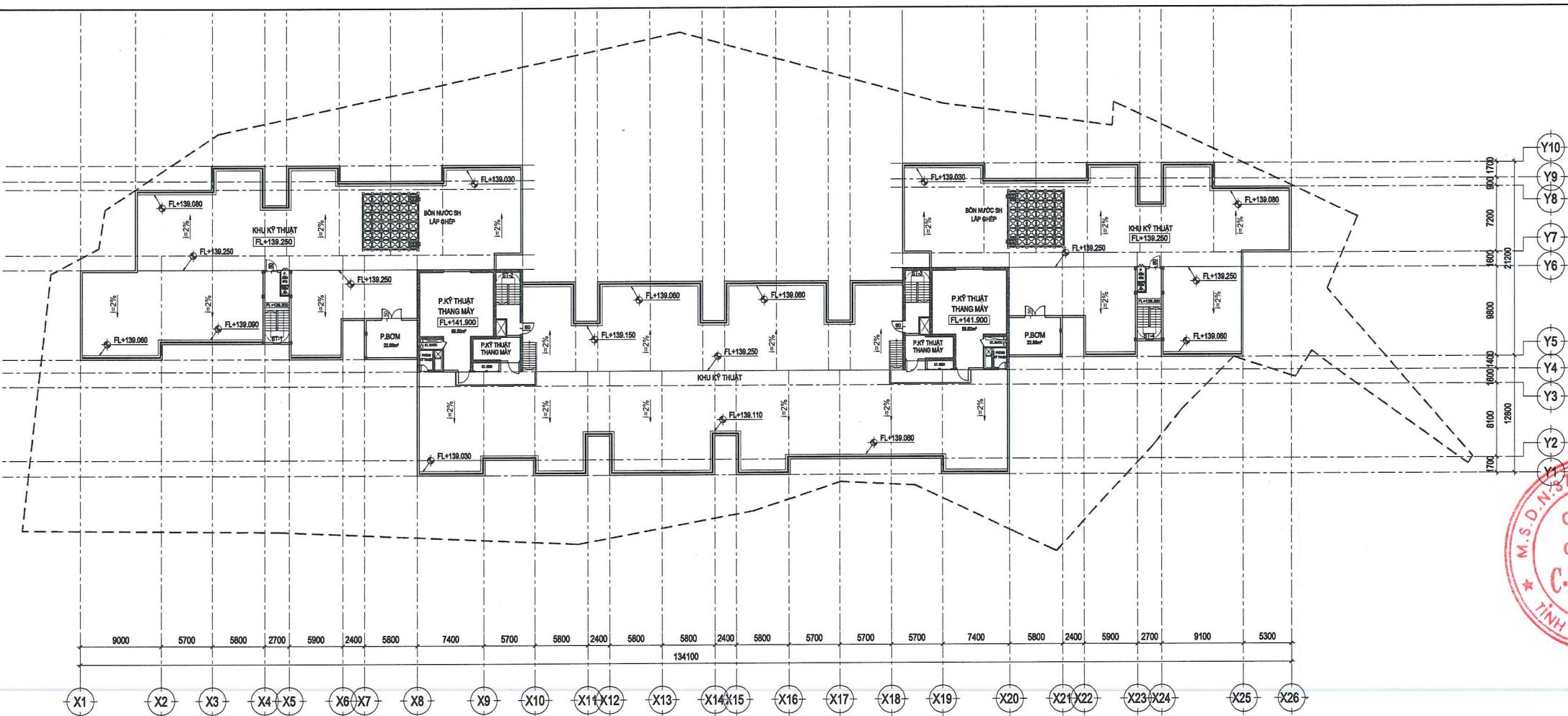
MẶT BẰNG TẦNG KỸ THUẬT TL: 1/300 DIỆN TÍCH SÀN: 366.74m²
