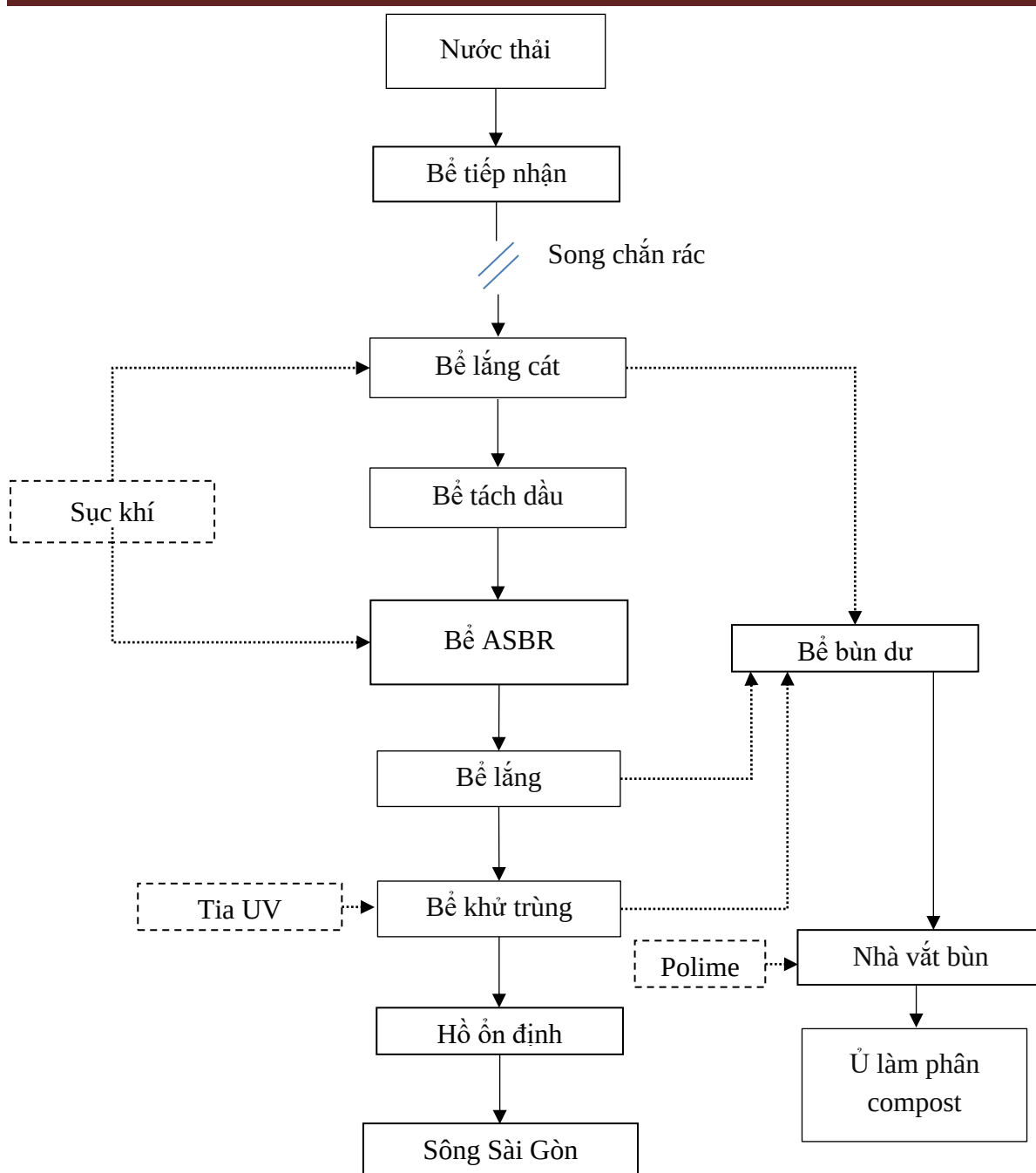
Hình 2.2. Quy trình công nghệ xử lý nước thải của nhà máy xử lý nước thải thành phố Thuận An
