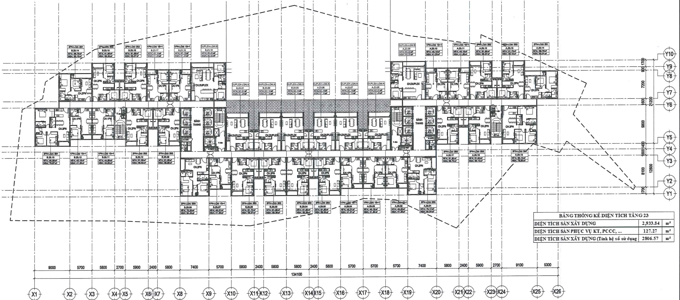
MẶT BẰNG TẦNG 23 TL: 1/300 DIỆN TÍCH SÀN: 2933.84m 2
