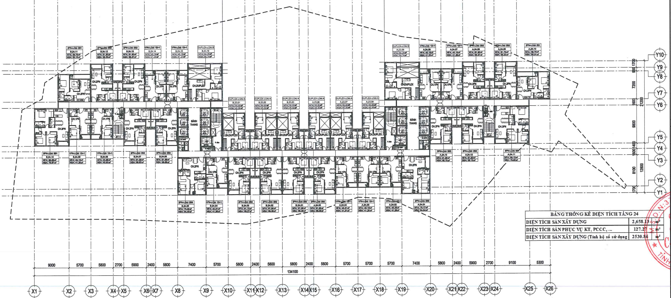
MẶT BẰNG TẦNG 24 TL: 1/300 DIỆN TÍCH SÀN: 2658.13m 2
