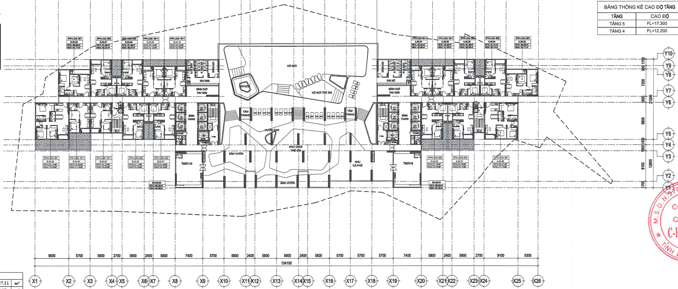
MẶT BẰNG TẦNG 5 TL: 1/300 DIỆN TÍCH SÀN: 3687.11 m 2
