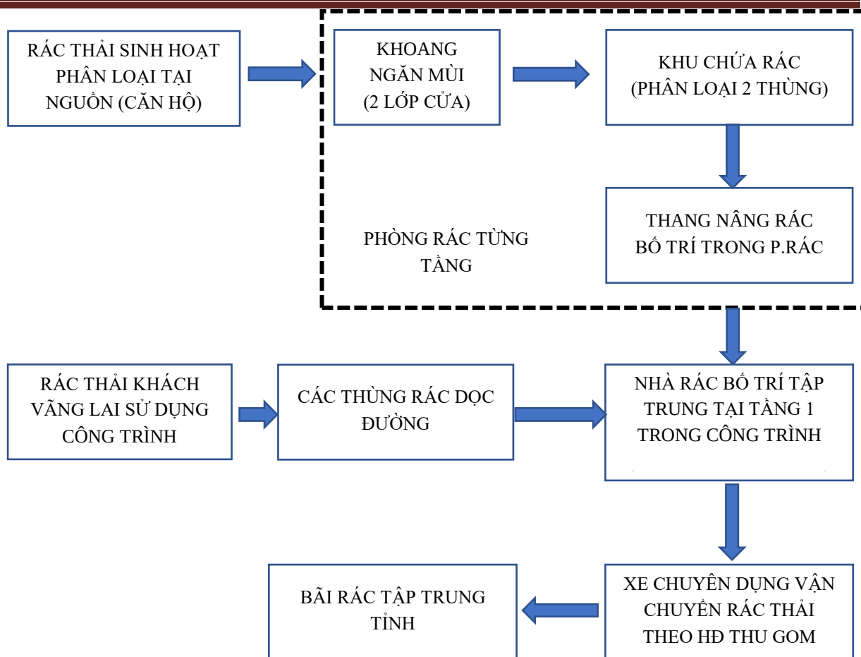
Hình 3.5. Sơ đồ thu gom rác tại dự án
