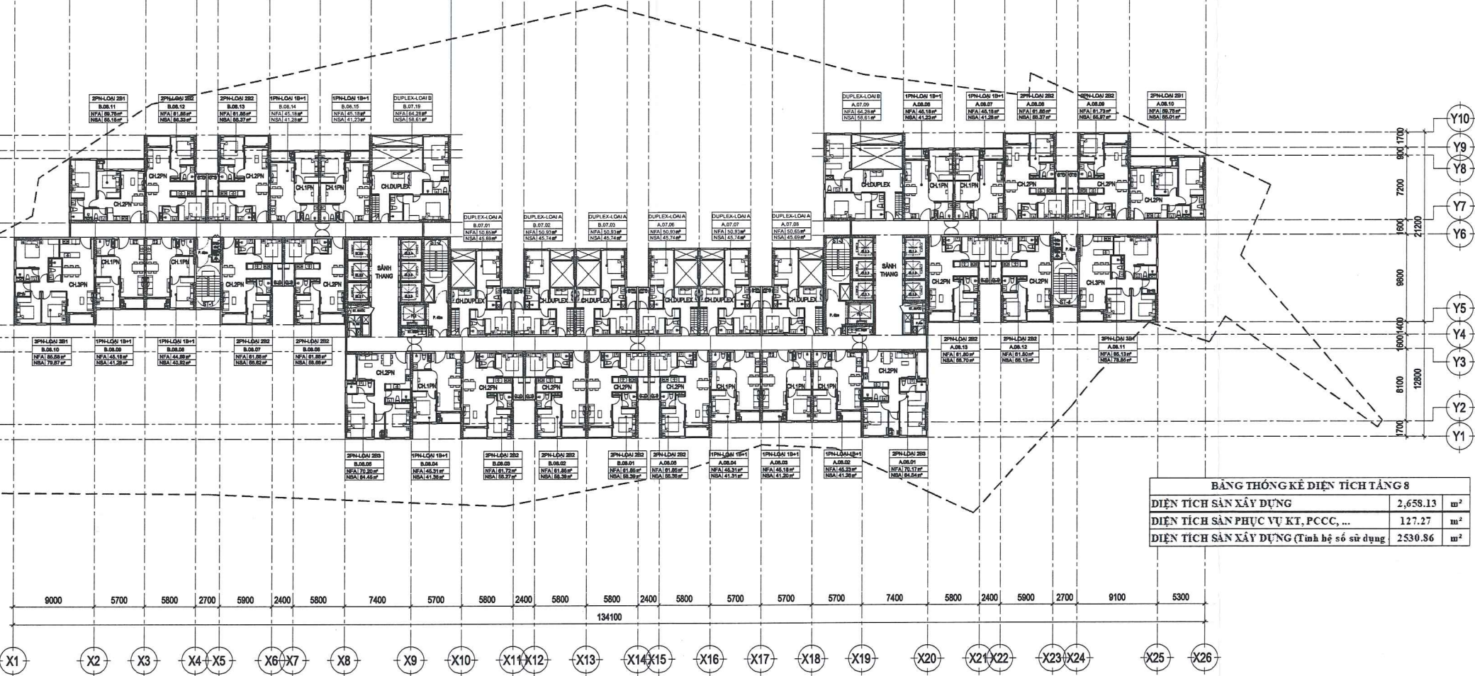
MẶT BẰNG TẦNG 8 TL: 1/300 DIỆN TÍCH SÀN: 2658.13m 2
