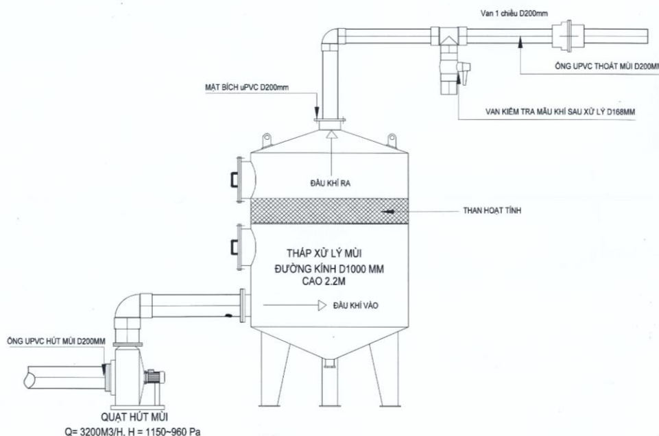
Hình 1.13. Hệ thống xử lý khí thải (mùi hôi) từ các cụm xử lý sơ bộ
