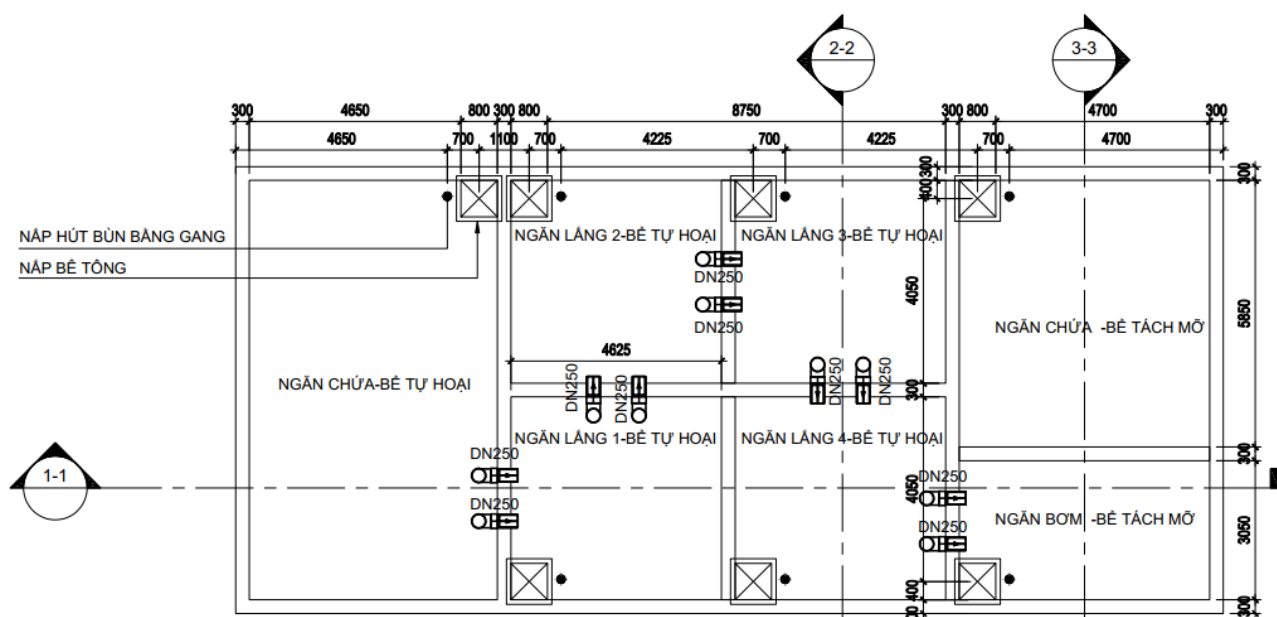
Hình 3.4. Sơ đồ cấu tạo cụm bể tự hoại và bể tách mỡ
