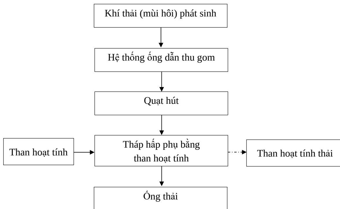
Hình. Quy trình xử lý mùi tại các cụm bể xử lý nước thải sơ bộ
