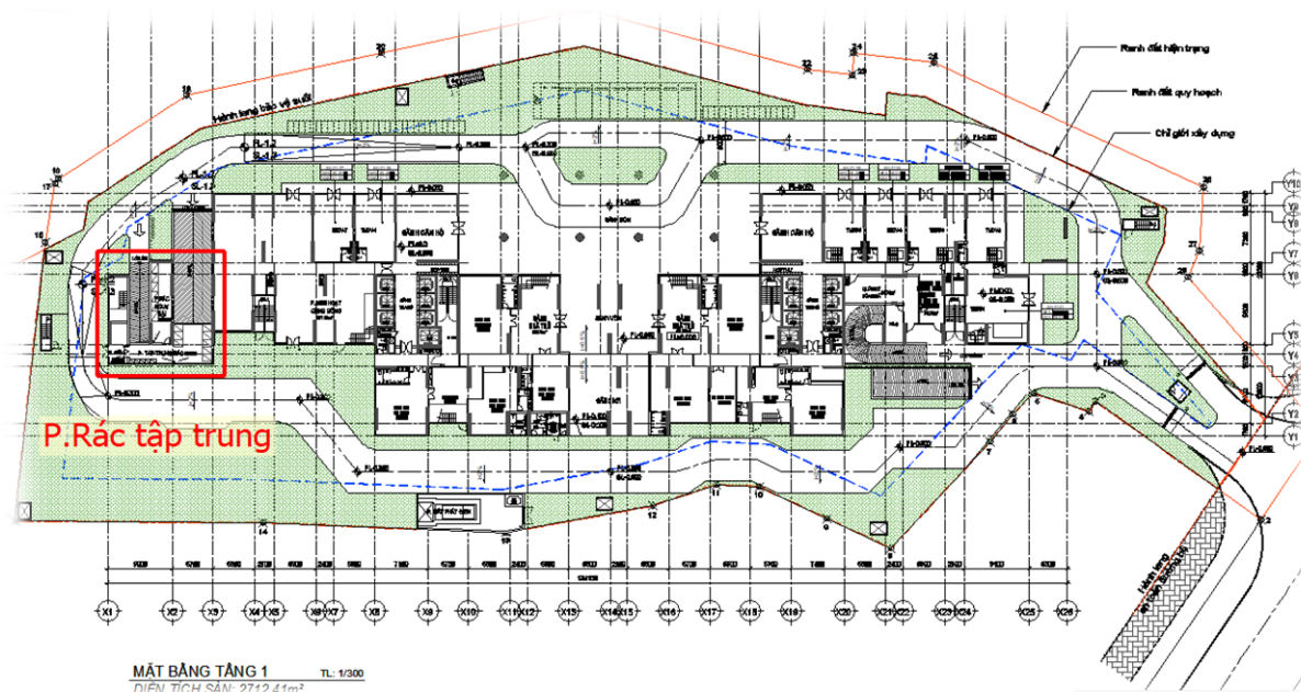
Bảng 3.6. Mặt bằng bố trí nhà rác tại dự án
