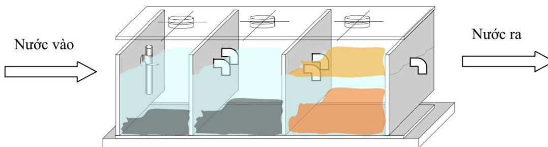
Hình 4-5. Cấu tạo bể tự hoại 3 ngăn
