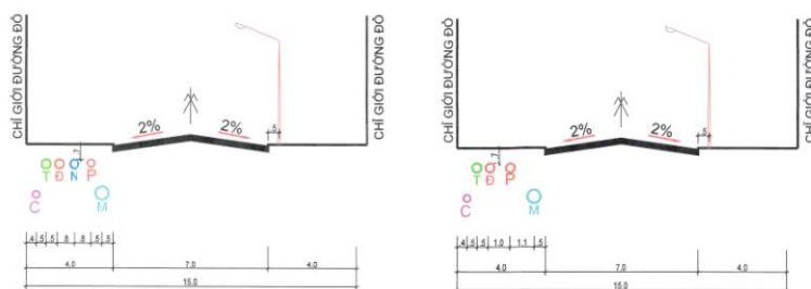
MẶT CẮT 2 - 2
