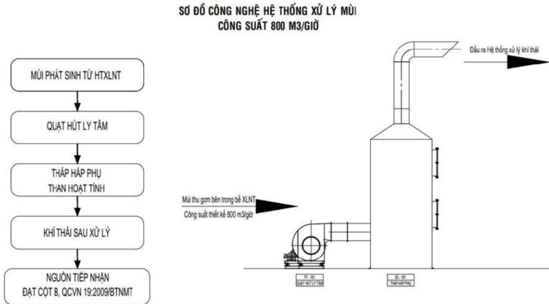
Hình 4-7. Sơ đồ hệ thống thoát xử lý mùi của HTXLNT của dự án
