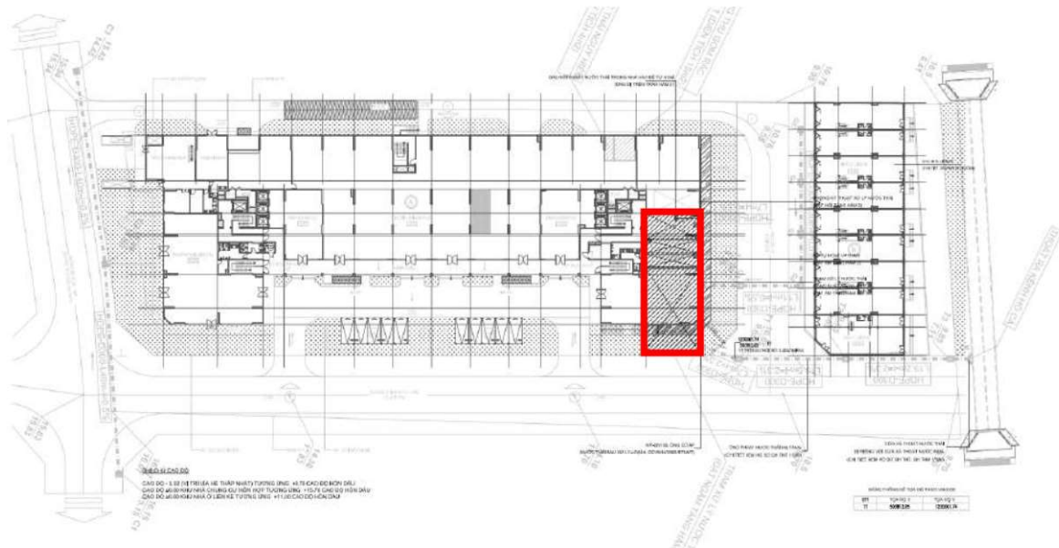
Hình 4-3. Vị trí trạm xử lý nước thải công suất 310 m 3 /ngày đêm
