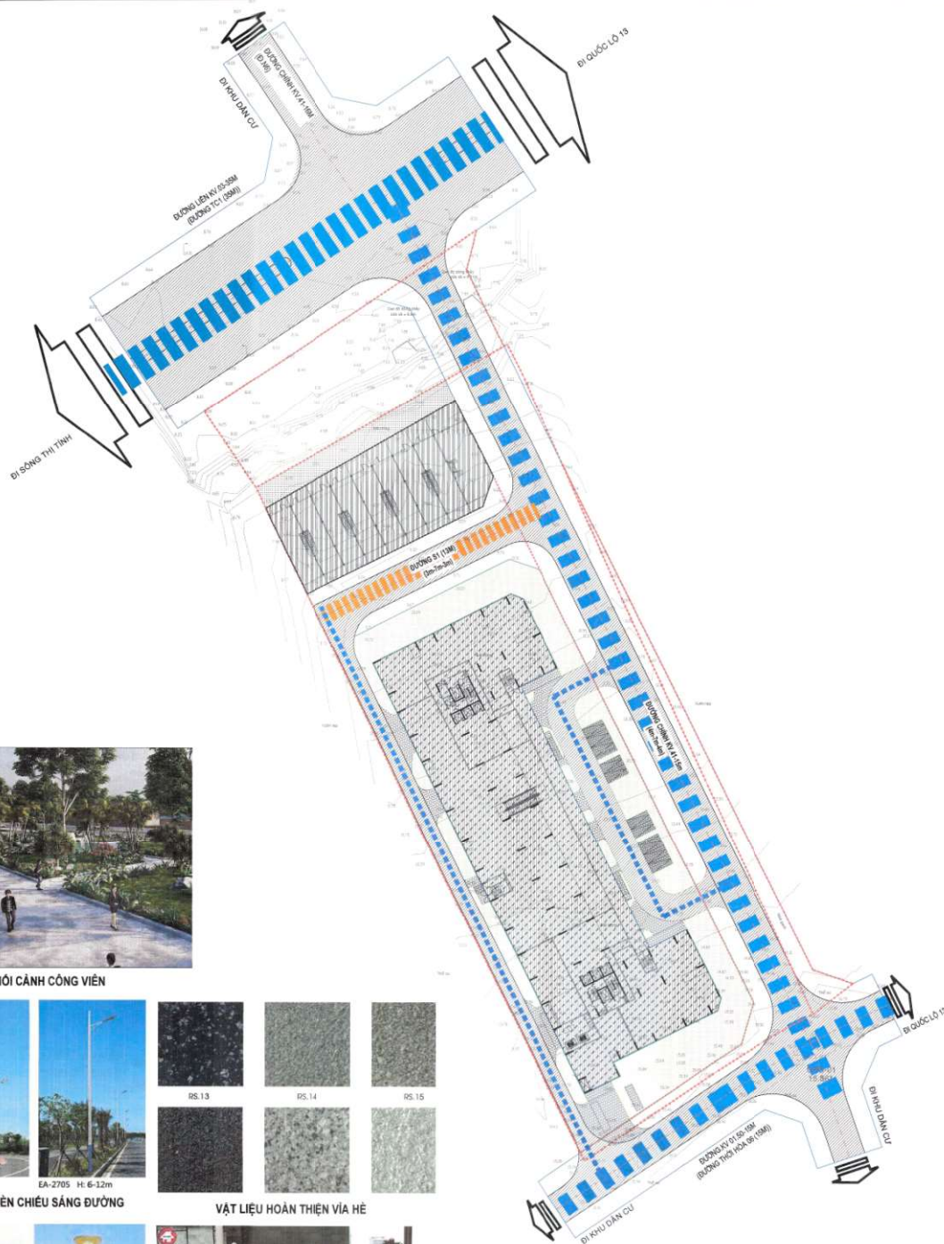
MẶT BẰNG TỔ CHỨC KHÔNG GIAN THIẾT KẾ ĐÔ THỊ
