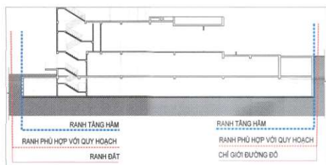
MẶT CẮT 1-1 TỈ LỆ 1/300
