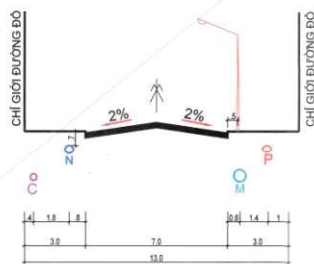
MẶT CẮT 1 - 1
