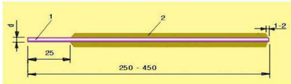
Hình 1-4. Cấu trúc que hàn
