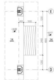
MẶT BẰNG RAM ĐỐC RD2 (TL:1/50)
