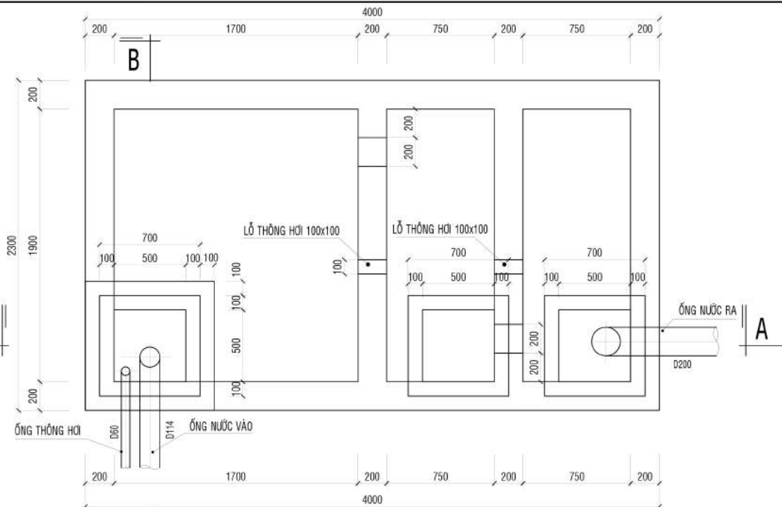
BỂ TỰ HOẠI 1
