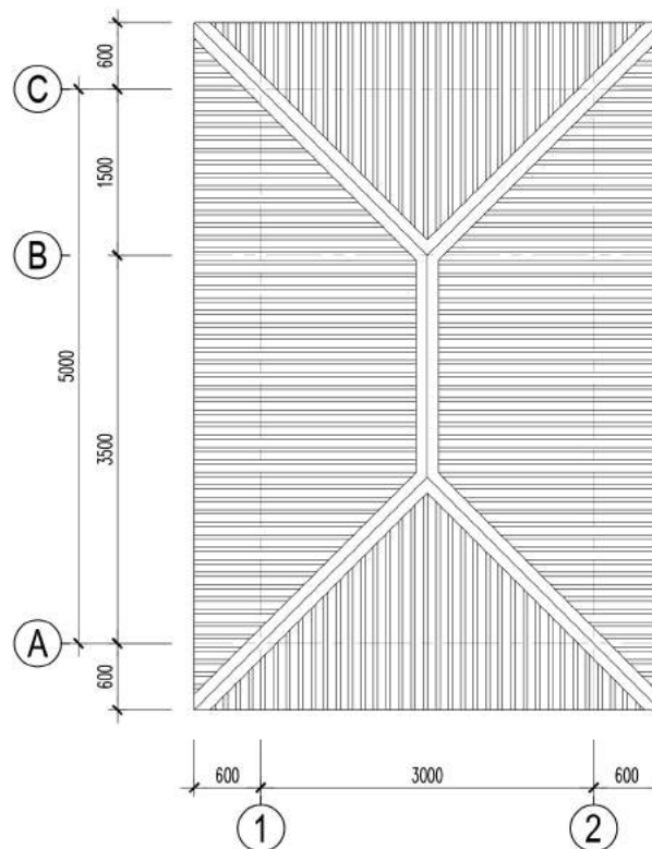
MẶT BẰNG MÁI T/L:1/100
