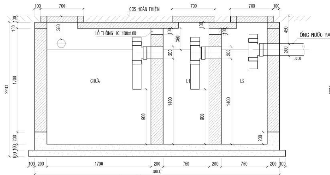
MẶT CẮT A - A TL 1/25
