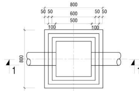
MẶT BẰNG HỒ GA
