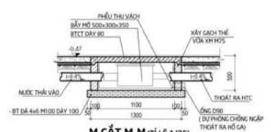
M.CẮT M-M (tỉ lệ 1/25)
