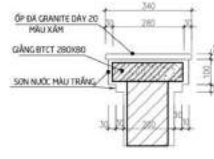
CẮT a-a (T.L: 1/10)
