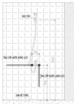
CHI TIẾT LẮP ĐẶT VỎ SEN
