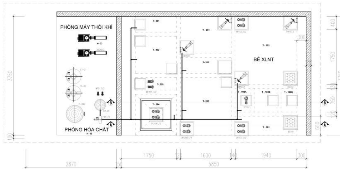
MẶT BẰNG BỐ TRÍ ỐNG THU GOM MÙI TỶ LỆ: 1/50
