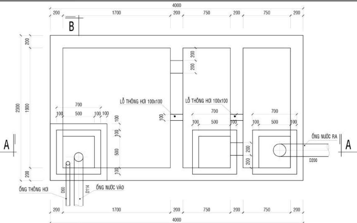
MẶT BẰNG BỂ TỰ HOẠI TL 1/25
