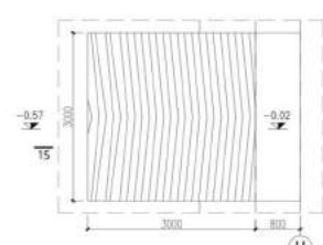
MẶT BẰNG RAM ĐỐC RD1 (TL:1/50)
