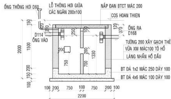
MẶT CẮT A-A TỶ LỆ: 1/50
