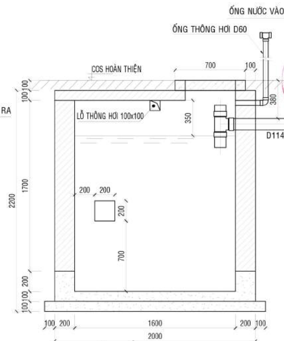
MẶT CẮT B - B TL 1/25
