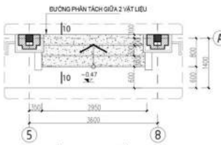
MẶT BẰNG TẦM CẤP TC2 (TL:1/50)
