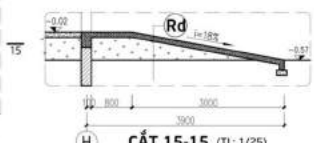
CẮT 15-15 (TL: 1/25)
