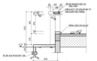
CẮT 12-12 (TL: 1/25)
