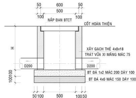
MẶT CẮT 1-1 TỶ LỆ: 1/20
