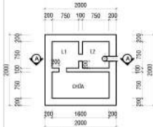
MẶT BẰNG BỂ TỰ HOẠI
