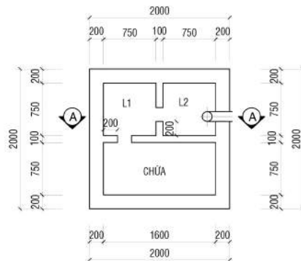
MẶT BẰNG BỂ TỰ HOẠI TỶ LỆ: 1/50
