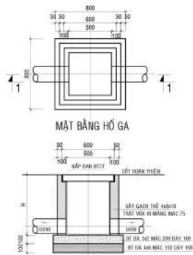
MẶT BẰNG HỒ GA
