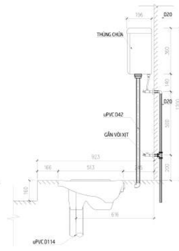
MẶT CẮT R-R
