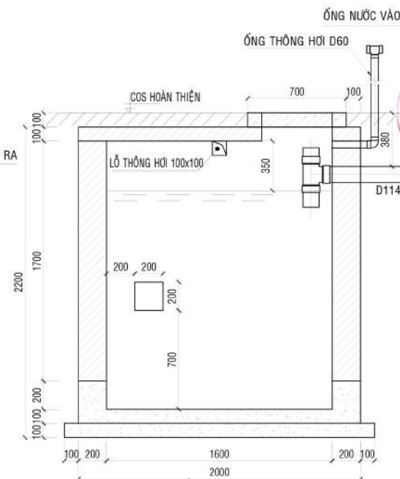
MẶT CẮT B - B TL 1/25
