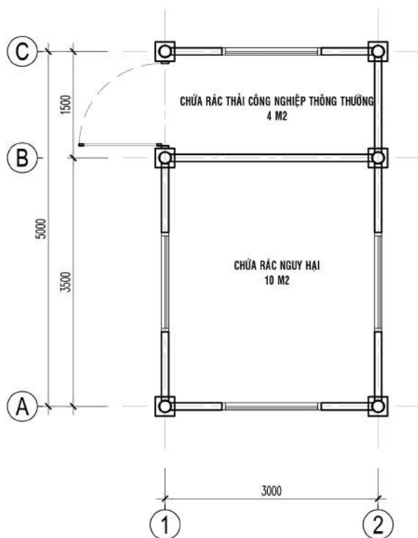
MẶT BẰNG T/L:1/100
