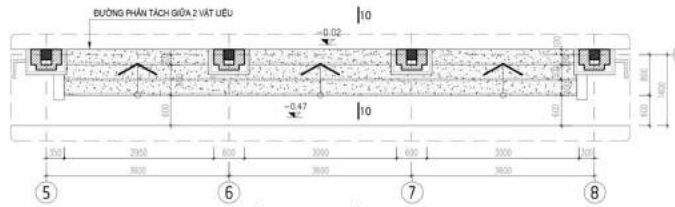
MẶT BẰNG TẦM CẤP TC1 (TL:1/50)
