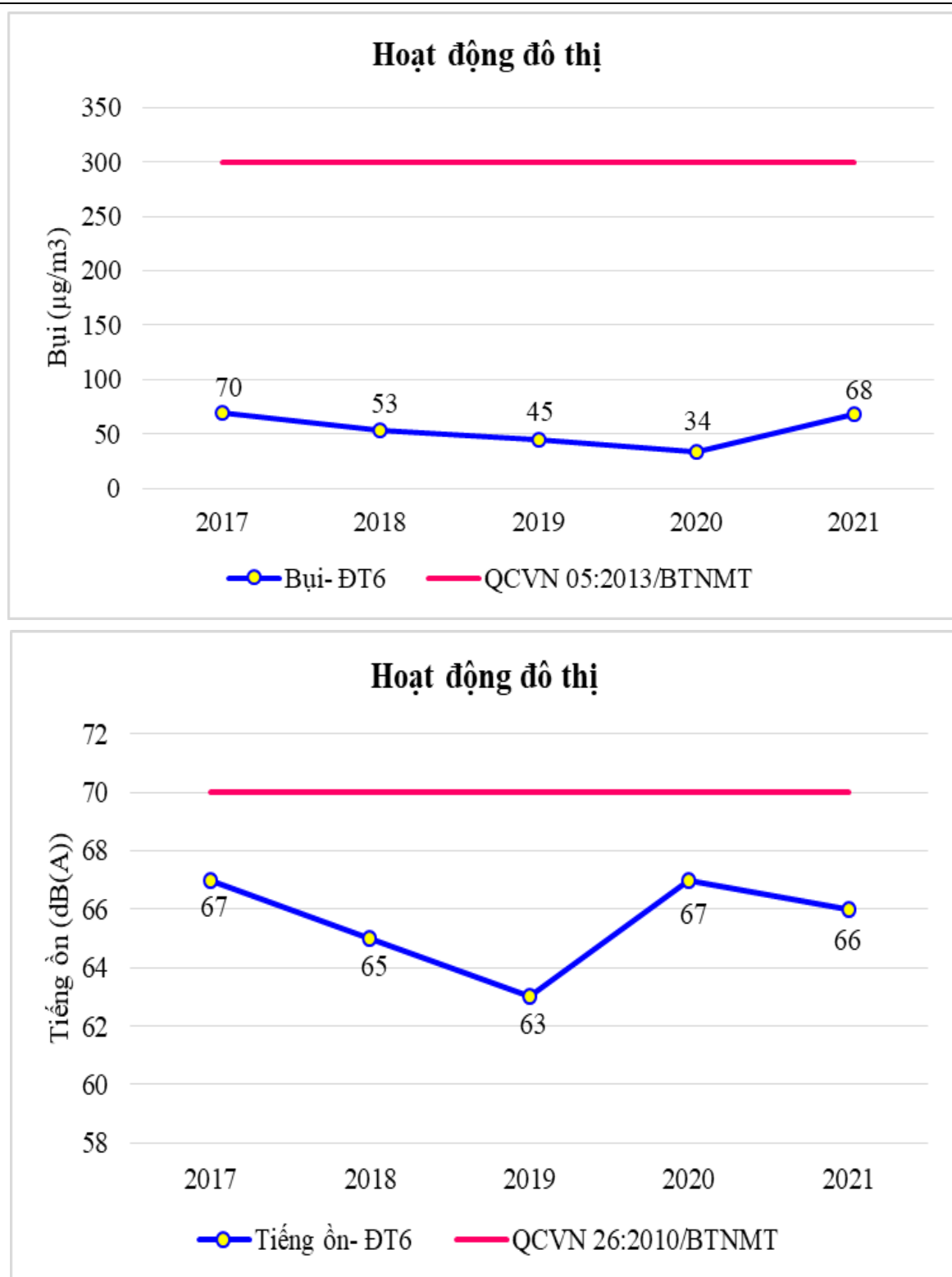
Biểu đồ 3.2. Diễn biến nồng độ bụi và tiếng ồn tại khu vực hoạt động đô thị
