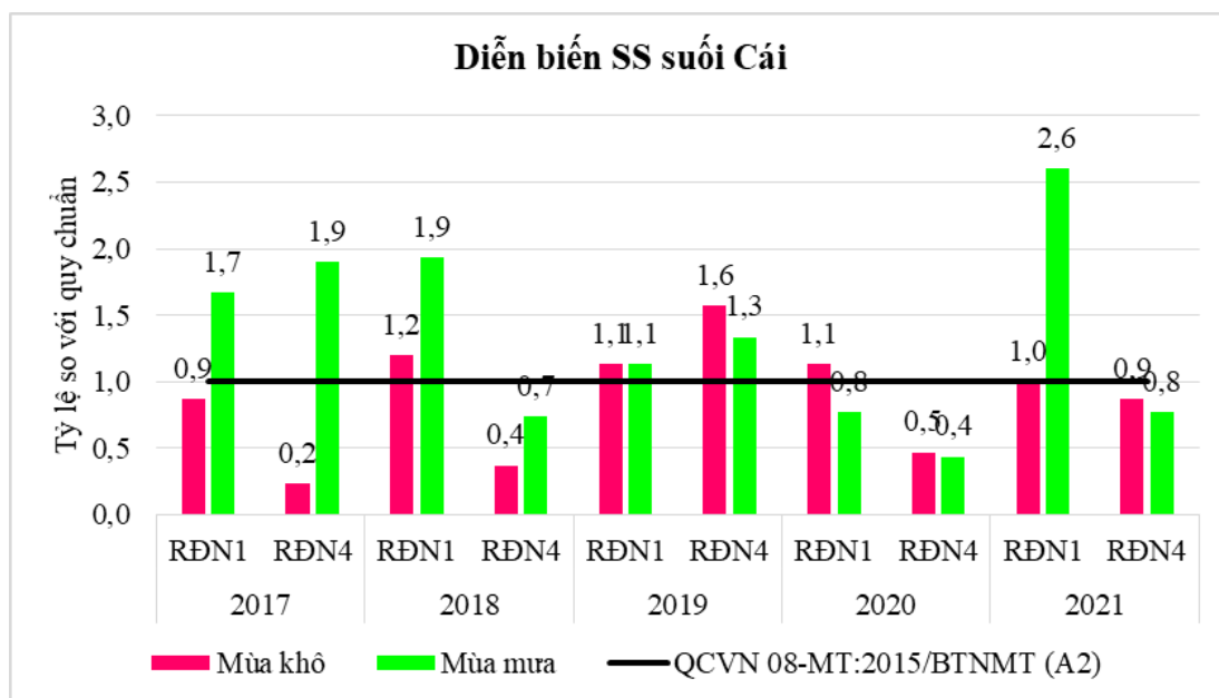
Hình 3.7: Biểu đồ Diễn biến thông số SS của suối Cái giai đoạn 2017-2021
