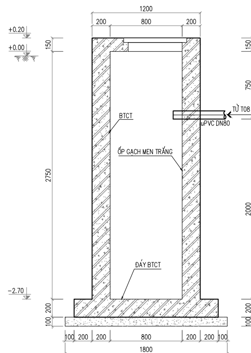
MẶT CẮT 2 - 2
