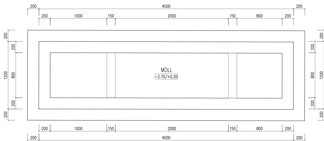
MẶT BẰNG ĐÁY MÁNG ĐO LƯU LƯỢNG
