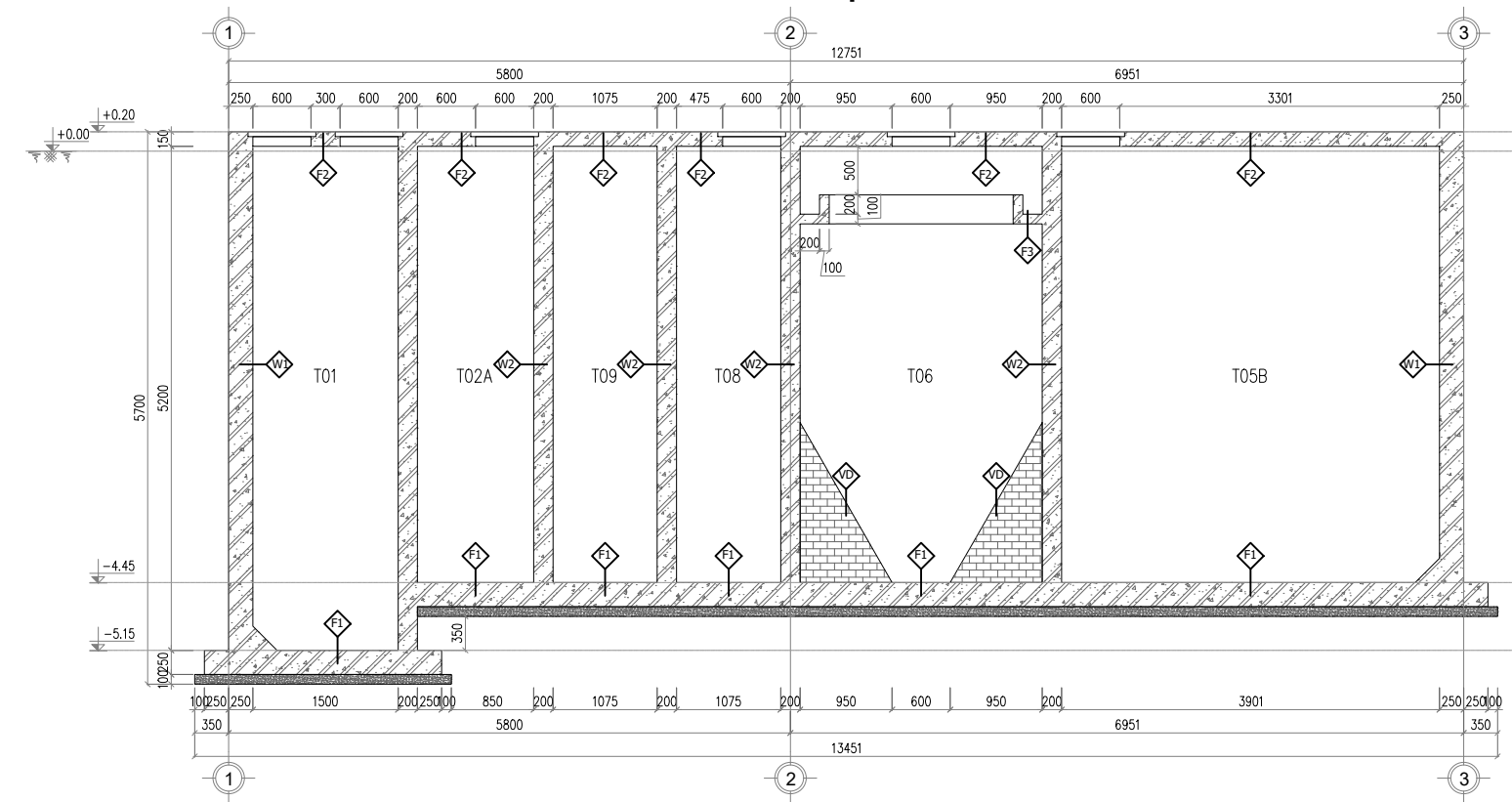
MẶT CẮT KIẾN TRÚC C - C
