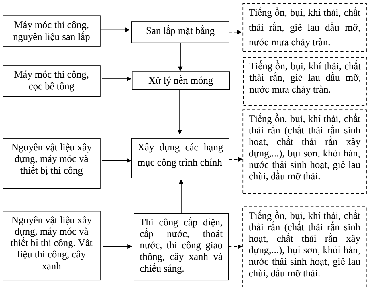
Hình 1.6. Sơ đồ thi công xây dựng dự án
