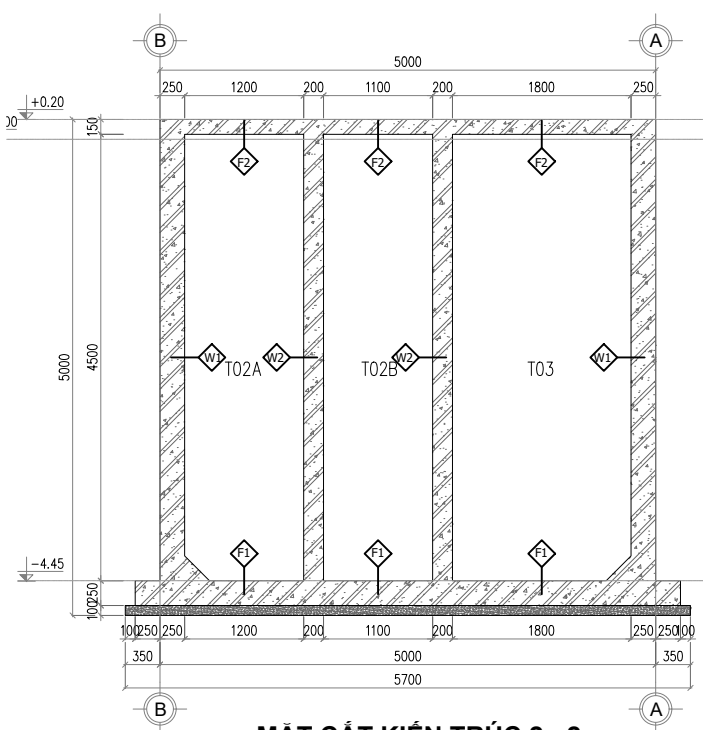
MẶT CẮT KIẾN TRÚC 2 - 2
