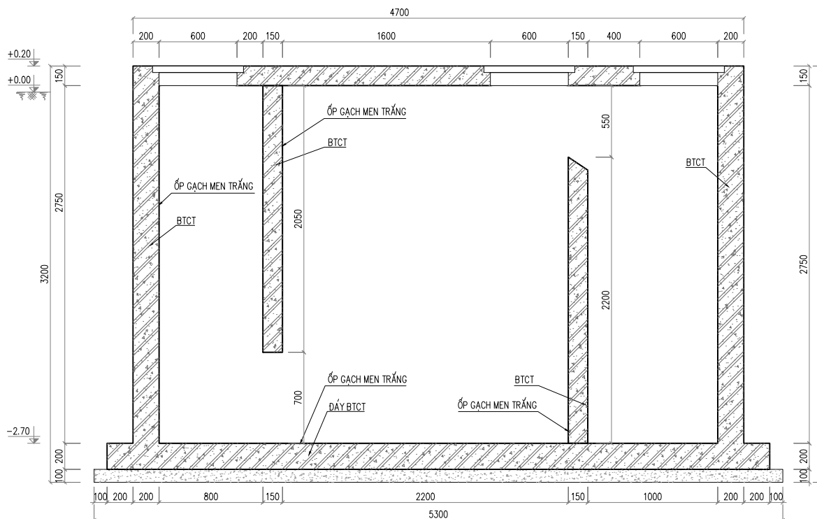
MẶT CẮT A - A
