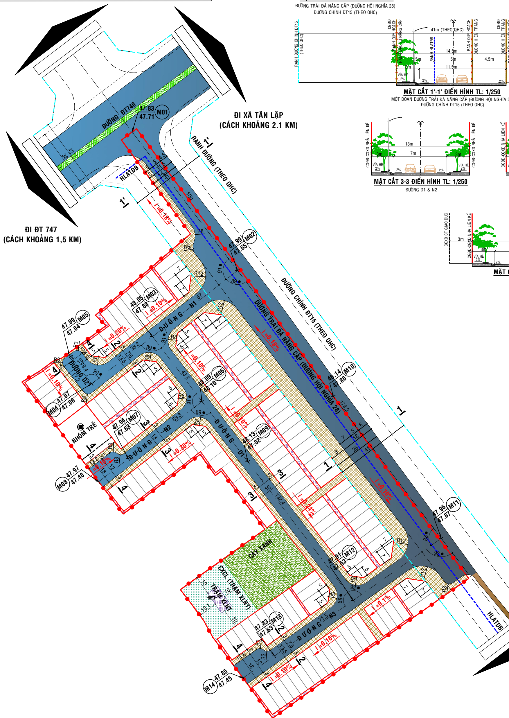
ĐƯỜNG CỤT D2, N2 &amp; N3
