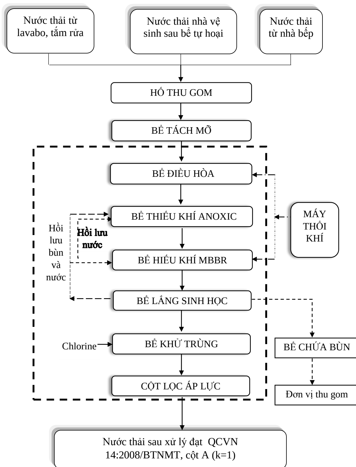
Hình 4.5. Sơ đồ quy trình công nghệ xử lý nước thải
