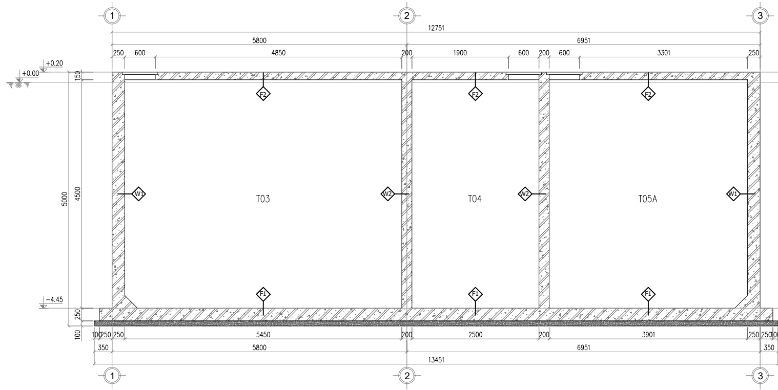
MẶT CẮT KIẾN TRÚC A - A
