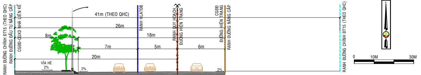
ĐƯỜNG TRẢI ĐÁ NÂNG CẤP (ĐƯỜNG HỘI NGHĨA 28) ĐƯỜNG CHÍNH ĐT15 (THEO QHC)
