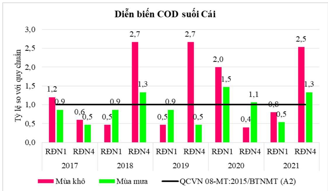
Hình 3.6: Biểu đồ diễn biến thông số COD của suối Cái giai đoạn 2017-2021
