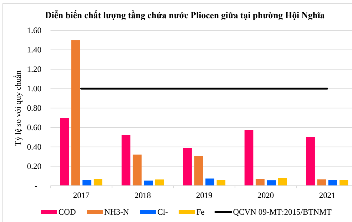
Hình 3.11: Biểu đồ diễn biến chất lượng nước dưới đất tại các tầng chứa nước của phường Hội Nghĩa trên địa bàn thị xã Tân Uyên giai đoạn 2017-2021
