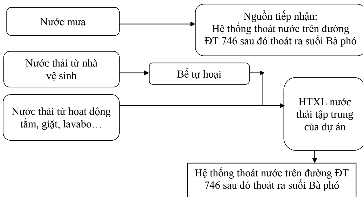
Hình 4.4. Sơ đồ thu gom và thoát nước mưa, nước thải tại dự án
