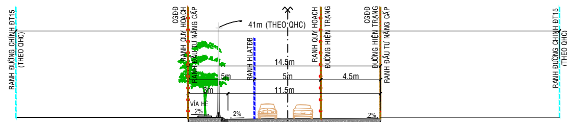
ĐƯỜNG TRẢI ĐÁ NÂNG CẤP (ĐƯỜNG HỘI NGHĨA 28) ĐƯỜNG CHÍNH ĐT15 (THEO QHC)
