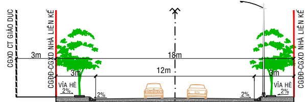
ĐƯỜNG CỤT D2, N2 & N3
