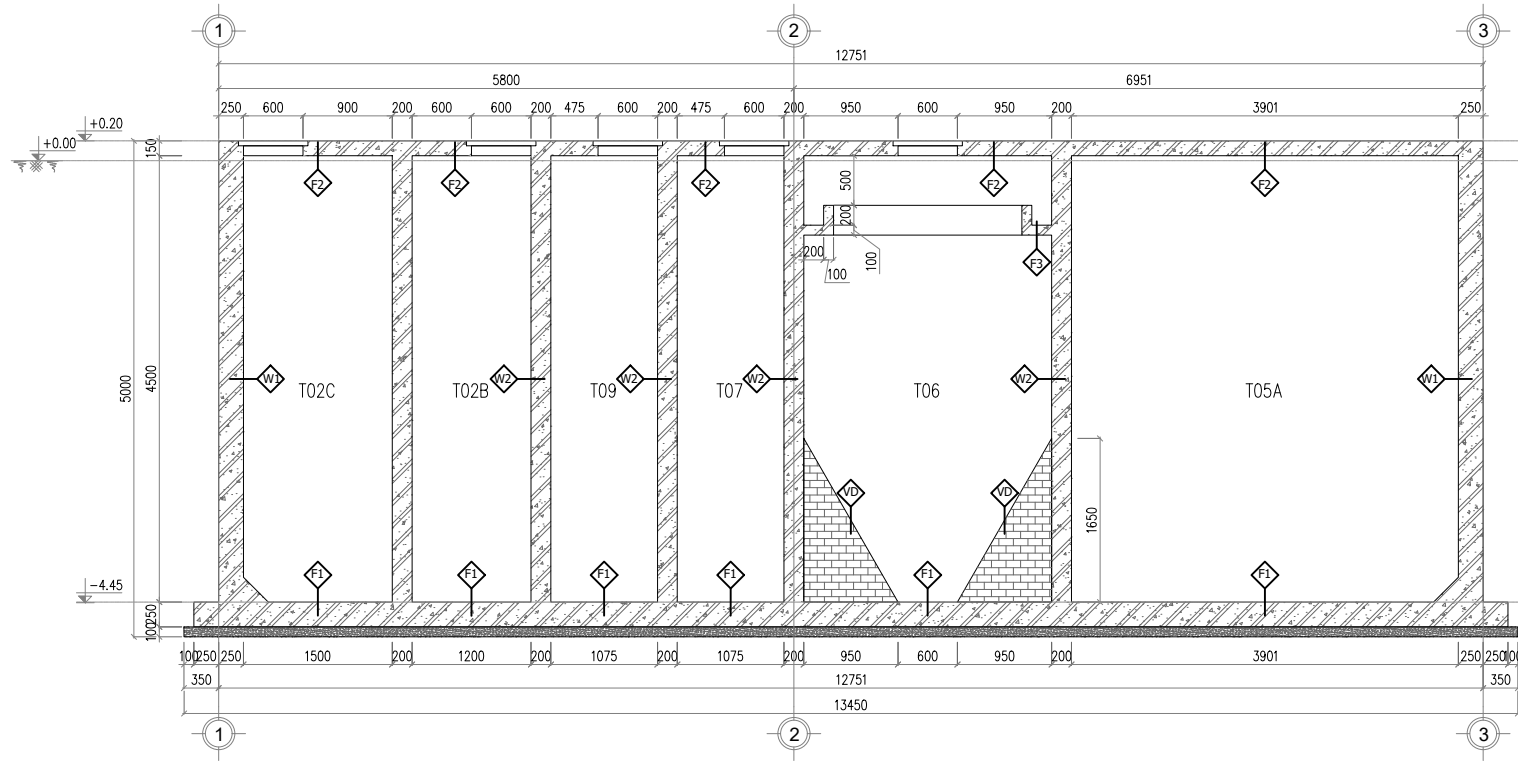
MẶT CẮT KIẾN TRÚC B - B
