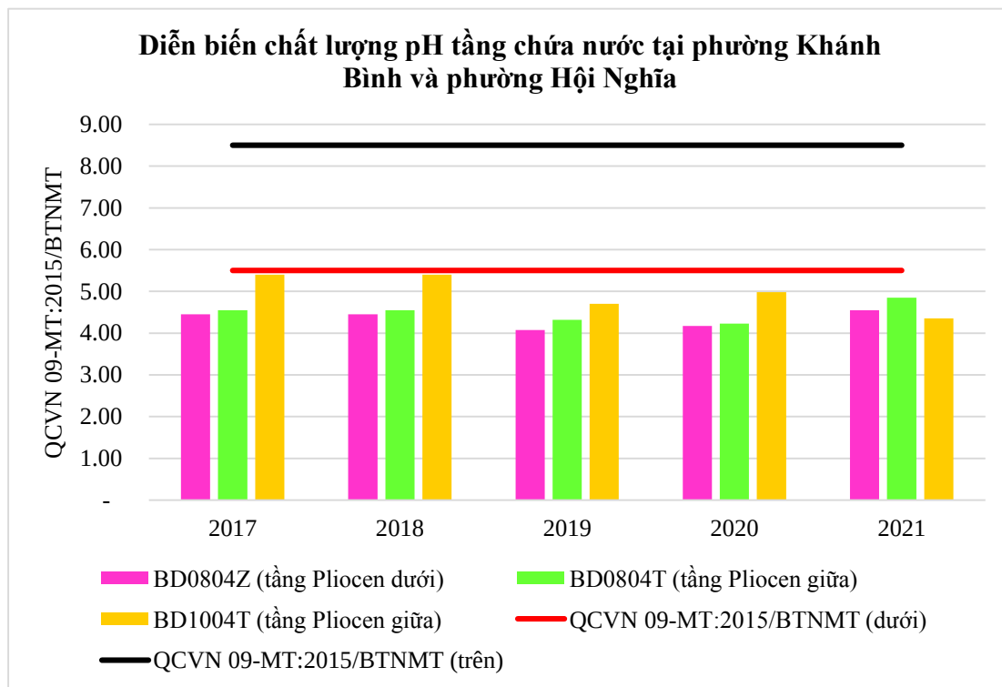
Hình 3.10: Biểu đồ diễn biến pH tại các tầng chứa nước khu vực phường Khánh Bình và phường Hội Nghĩa giai đoạn 2017-2021
