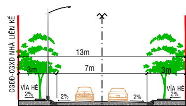
ĐƯỜNG D1 &amp; N2
