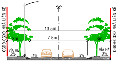
ĐƯỜNG N1 &amp; ĐƯỜNG N3
