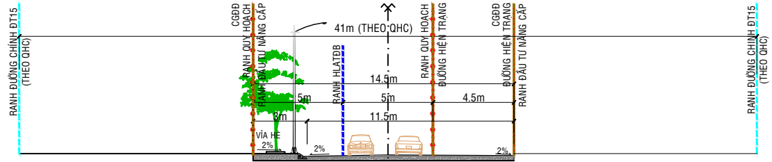
MỘT ĐOẠN ĐƯỜNG TRẢI ĐÁ NÂNG CẤP (ĐƯỜNG HỘI NGHĨA 28) ĐƯỜNG CHÍNH ĐT15 (THEO QHC)
