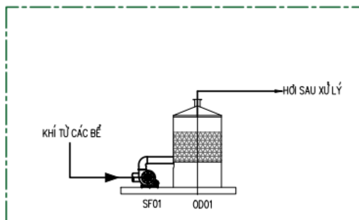
Hình 4.3: Tháp hấp phụ bằng than hoạt tính
