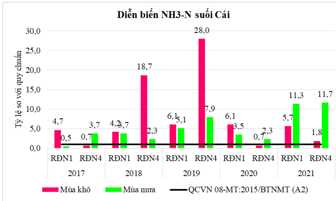
Biểu đồ 3.8 Diễn biến thông số NH 3 -N của suối Cái giai đoạn 2017-2021
