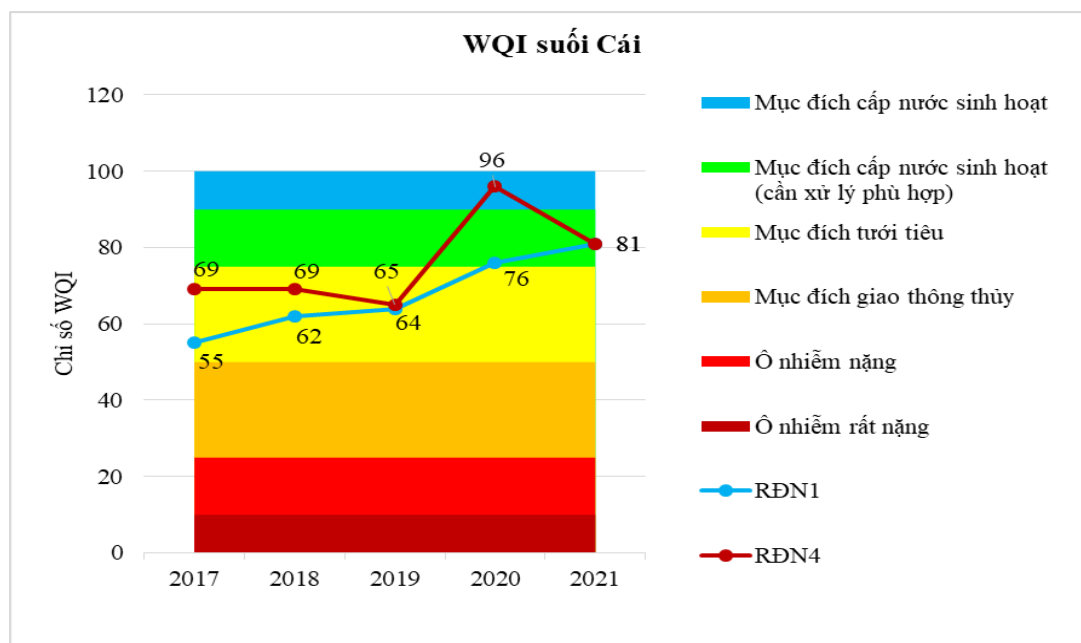
Hình 3.8: Biểu đồ chỉ số WQI nước mặt suối Cái giai đoạn 2017-2021
